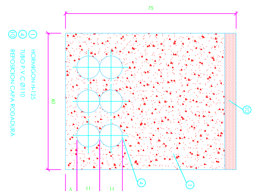
CANALIZACIONES CALZADA
